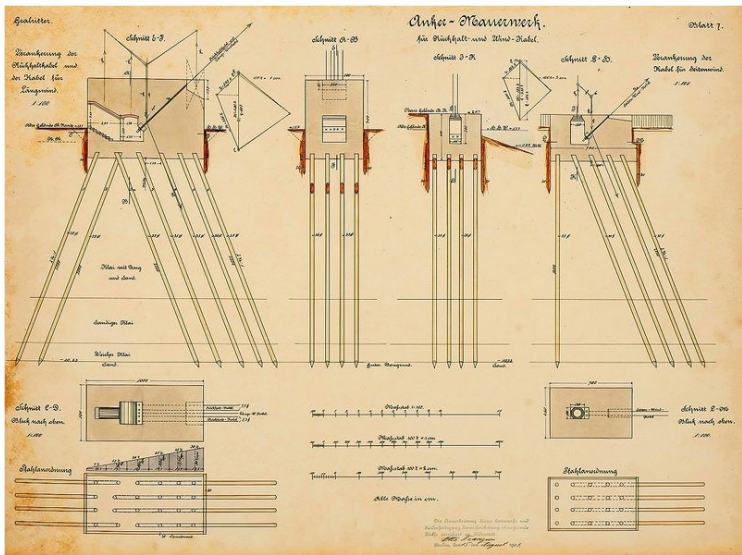
Abb. 6: Plan für die Gründung der Stützen.
