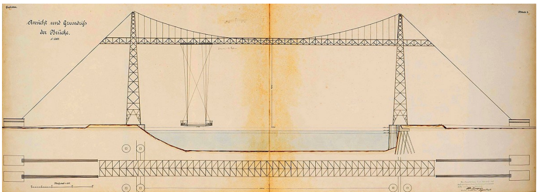
Abb. 4: Tragkonstruktion mit Schwebefähre in der Ansicht..
