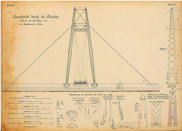
Abb. 5: Brückenquerschnitt und mit Kraftvektoren ermittelte Statik.
